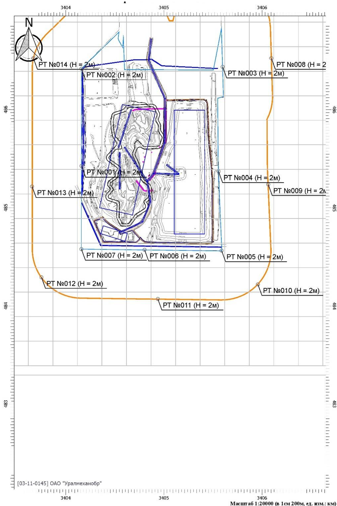
Рисунок 5 – Ситуационная карта-схема расположения объекта с санитарно-защитной зоной и расчетными точками
