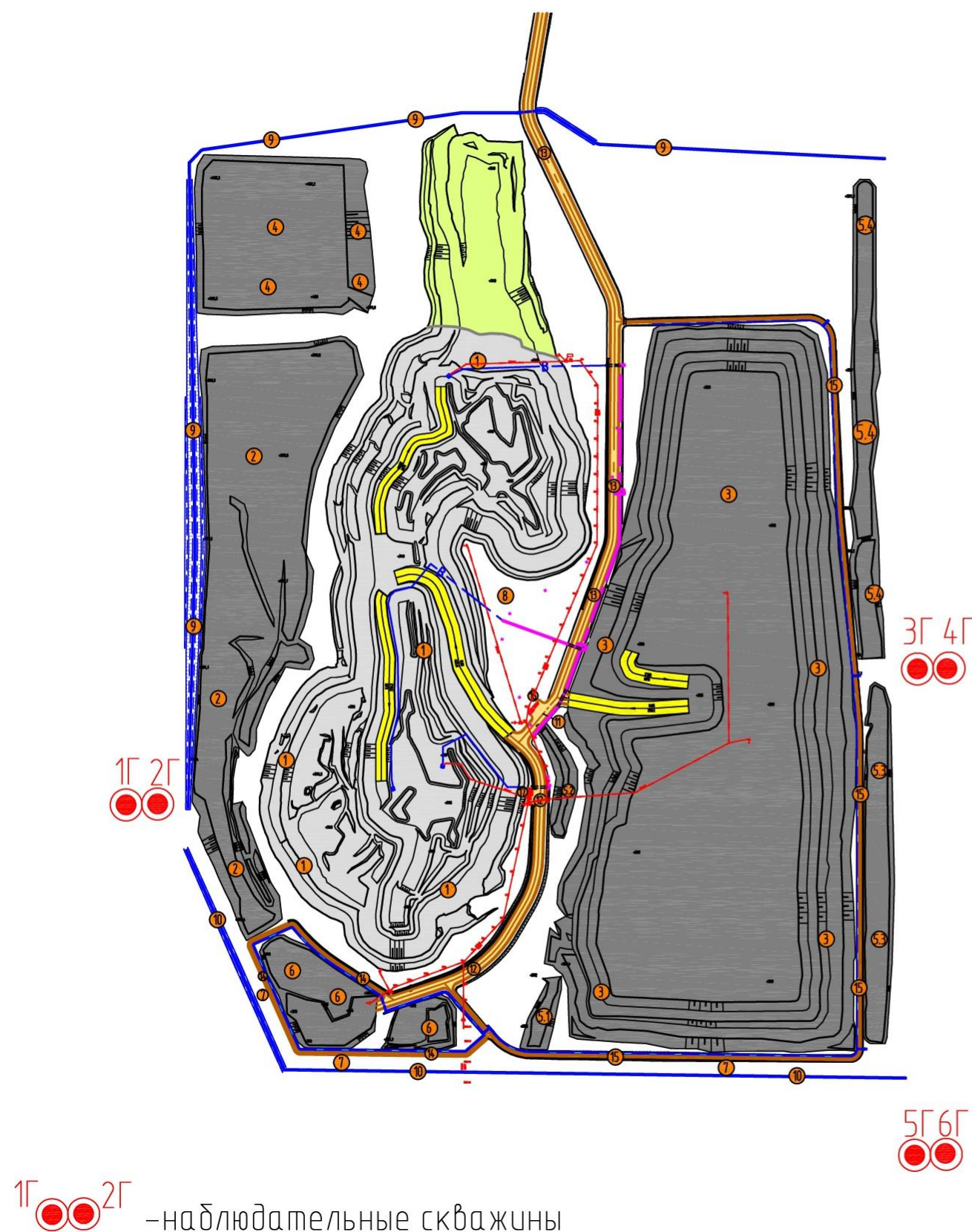
Рисунок 10 – Карта-схема расположения точек наблюдения за состоянием подземных вод
