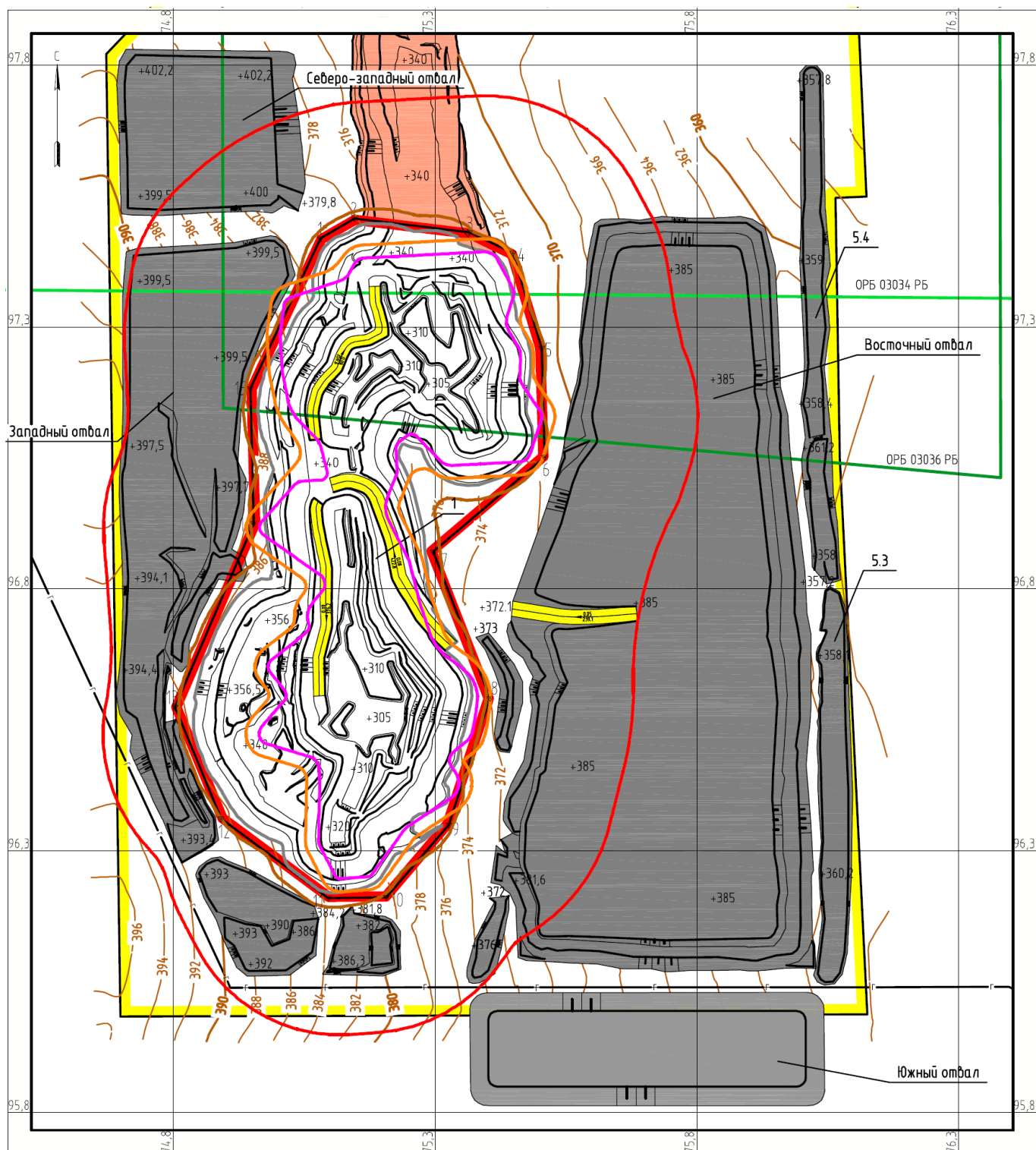
Рисунок 2 - План карьера и отвалов на конец разработки при альтернативном способе разработки
