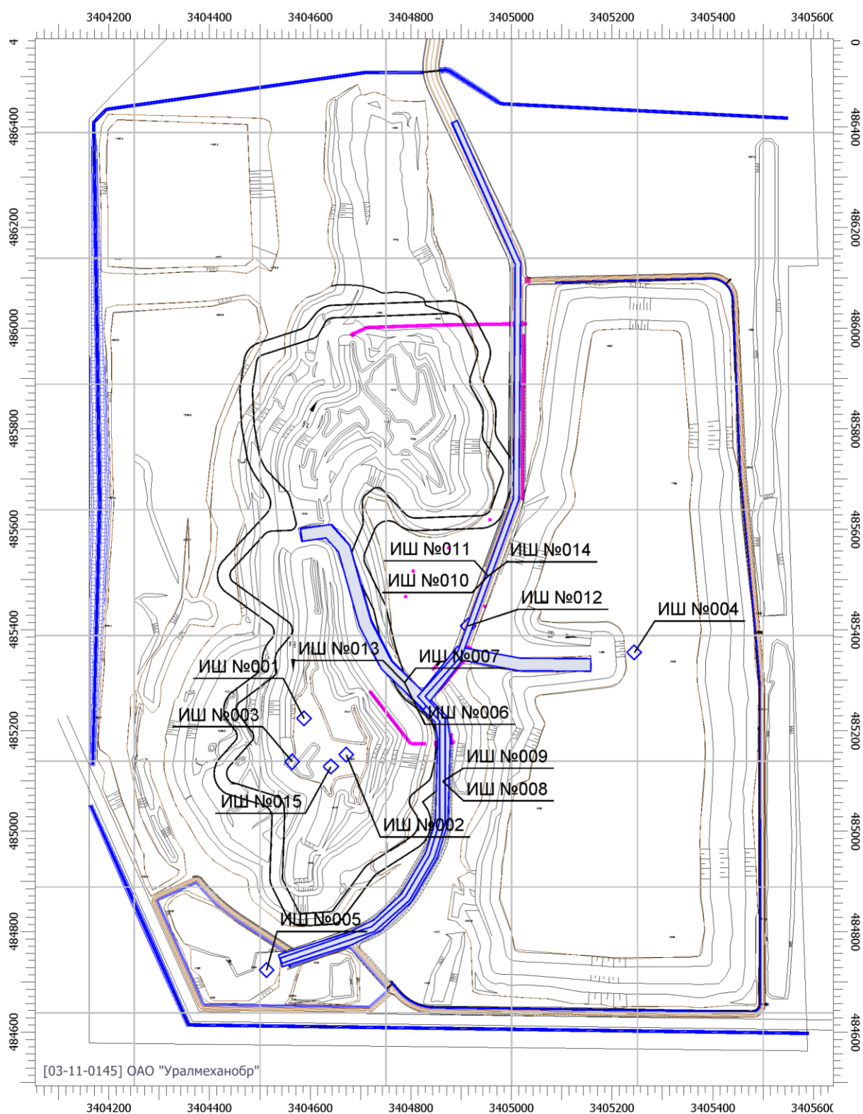
Рисунок 7 – Схема расположения источников шума Белозерского золоторудного месторождения ПАО «Гайский ГОК»
