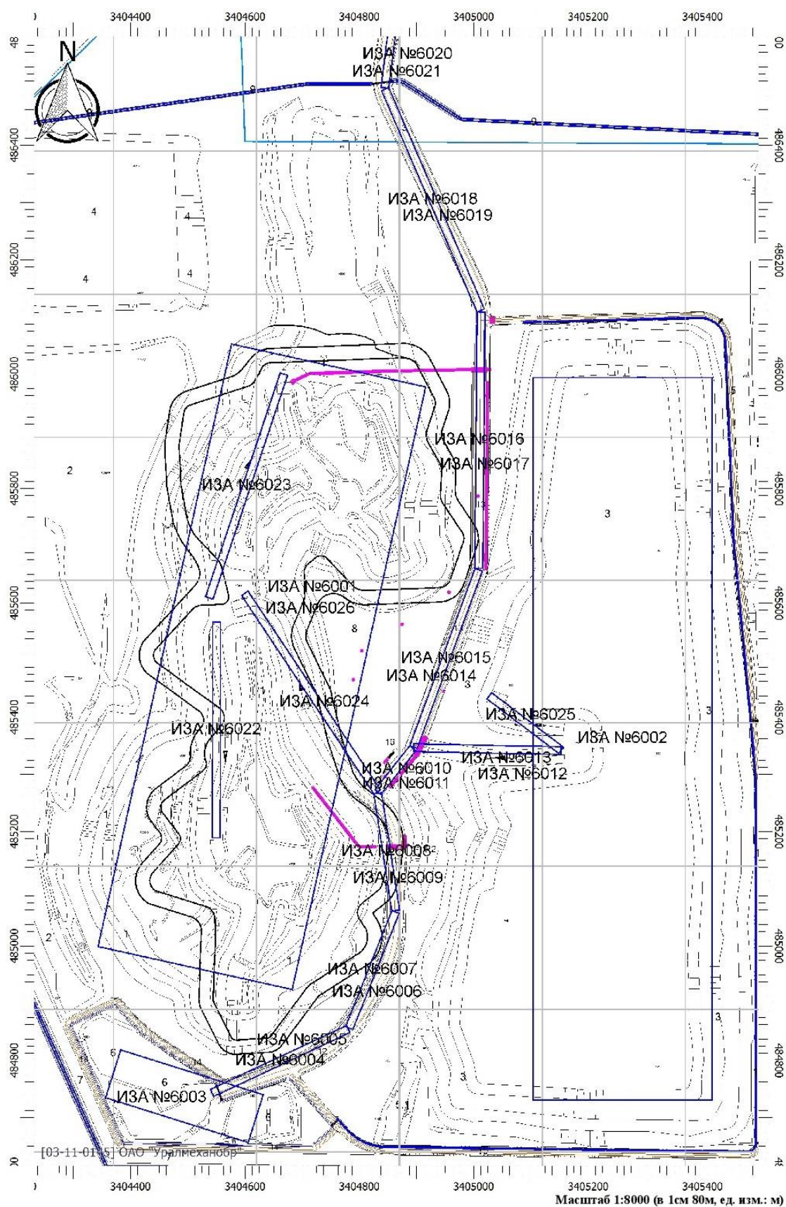
Рисунок 6 - Схема расположения источников выбросов загрязняющих веществ
